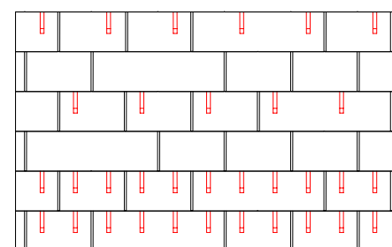
MONTÁŽNÍ SCHÉMA FX.12 1
