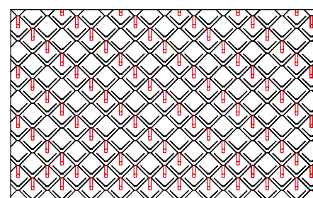
MONTÁŽNÍ SCHÉMA R2
