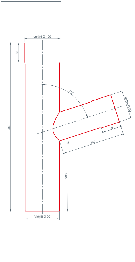
Odbočka kruhového svodu 100x80
