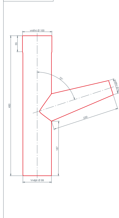
Odbočka kruhového svodu 100x50/75
