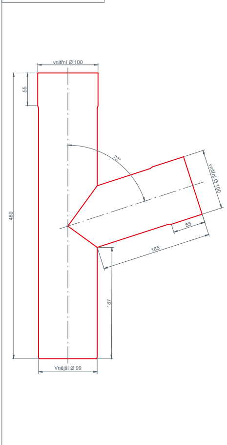
Odbočka kruhového svodu 100x100
