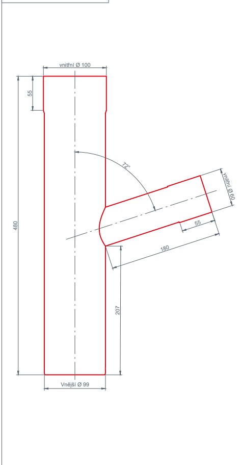
Odbočka kruhového svodu 100x60
